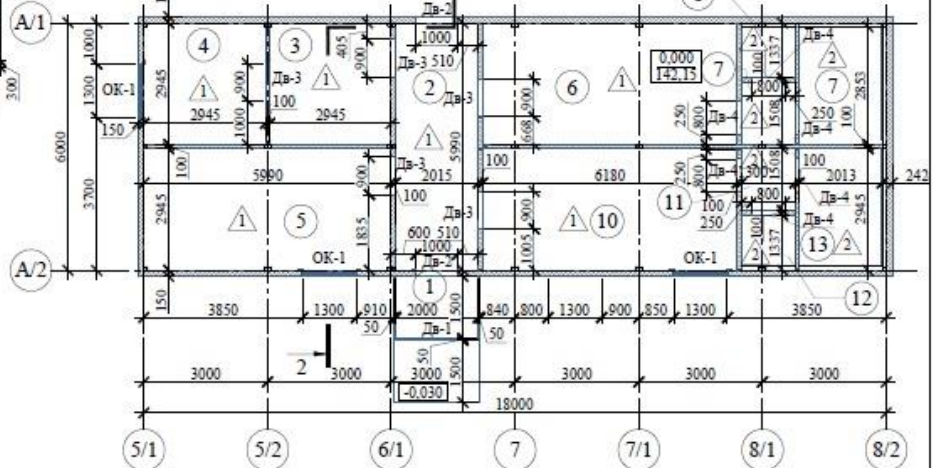
Монтажный план
