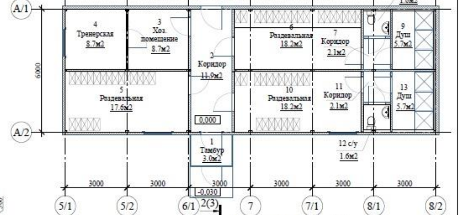
Монтажный план
