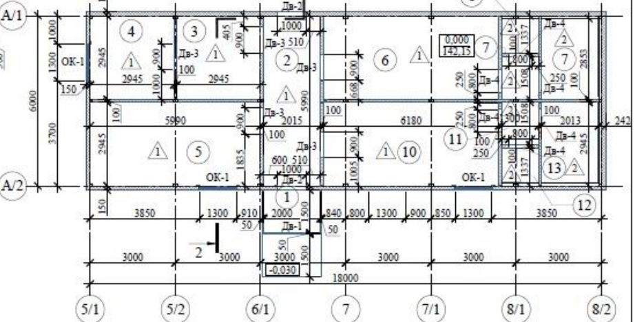
Монтажный план
