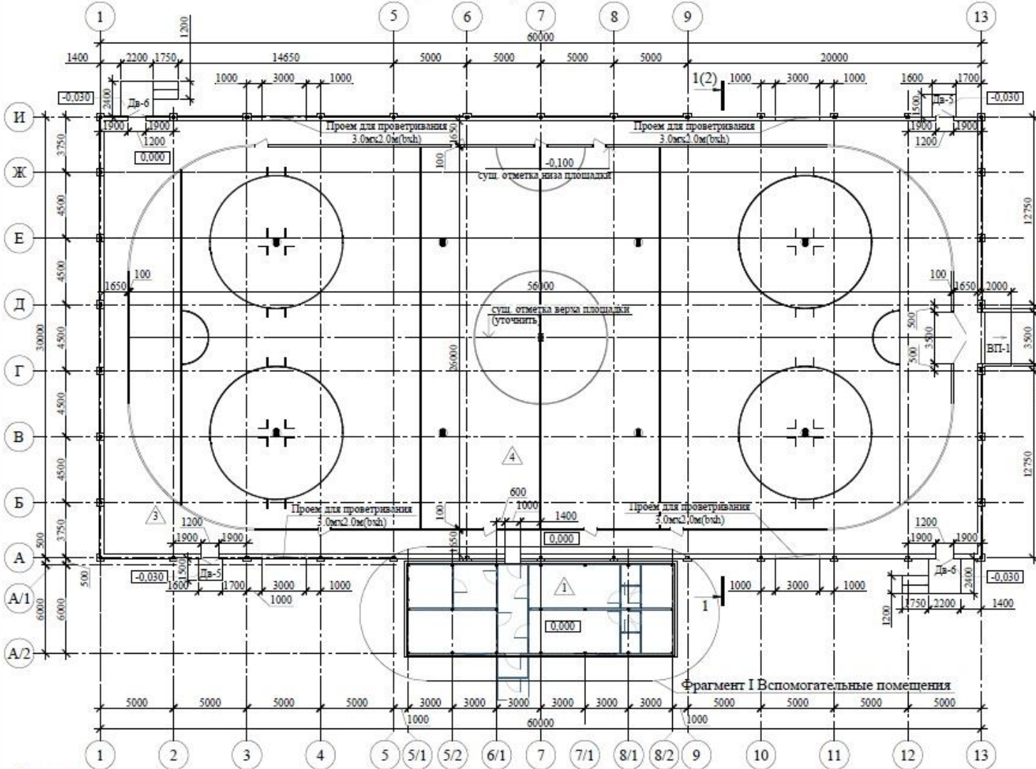
Общий план универсальной спортивной площадки
